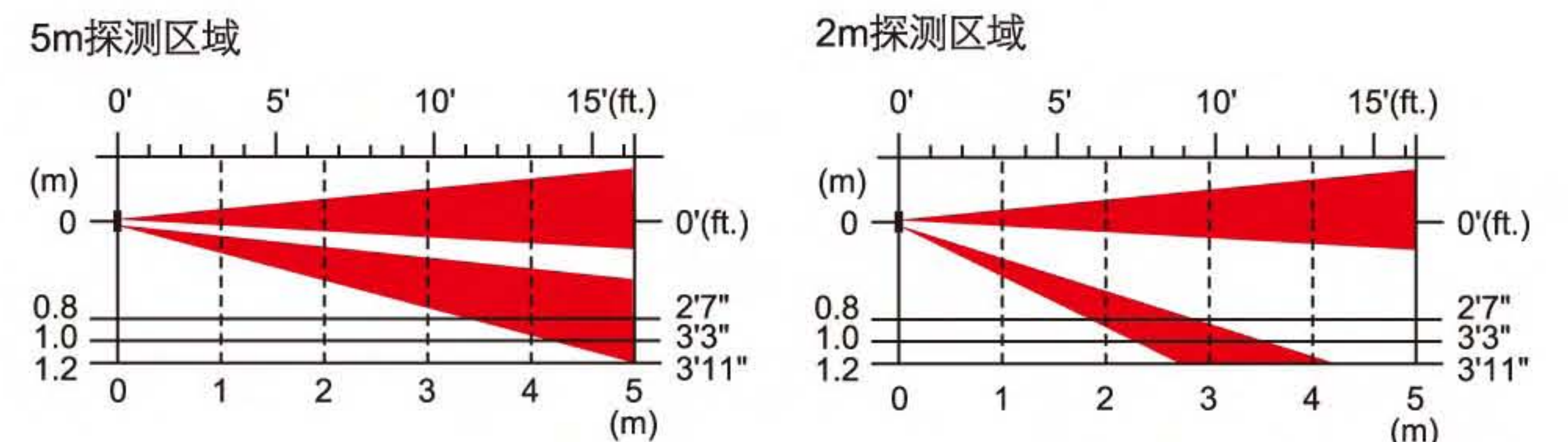
侧视图
